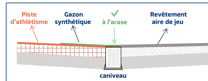
Plan de coupe
