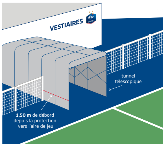
▶ Schémas n°32 : exemples de dispositifs de protection entre les vestiaires et le terrain
